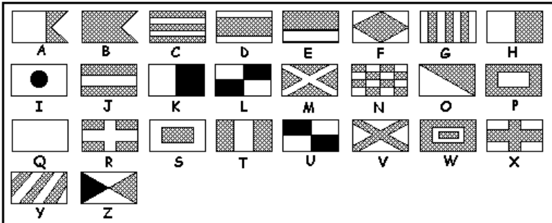
Illustration 1: Das Flaggenalphabet
