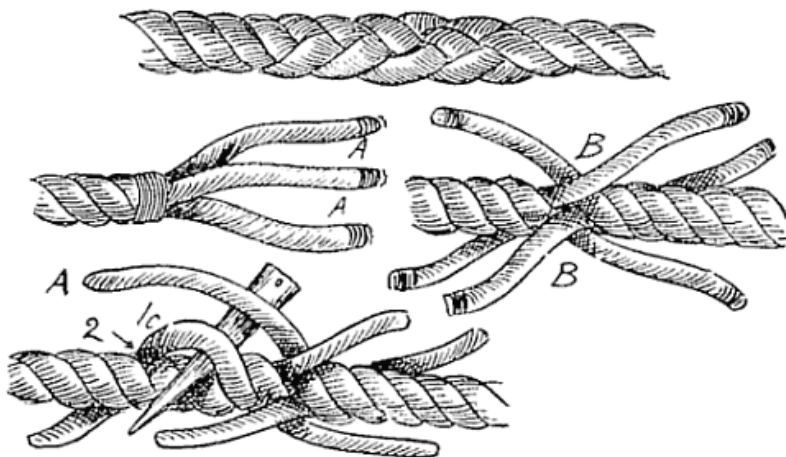
Illustration 12: Kurzspleiss in Arbeit
