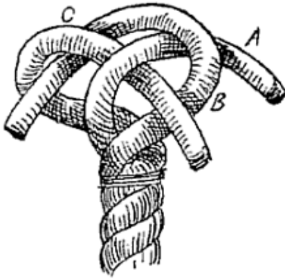
Illustration 8: Krone bei einem Endspleiss
